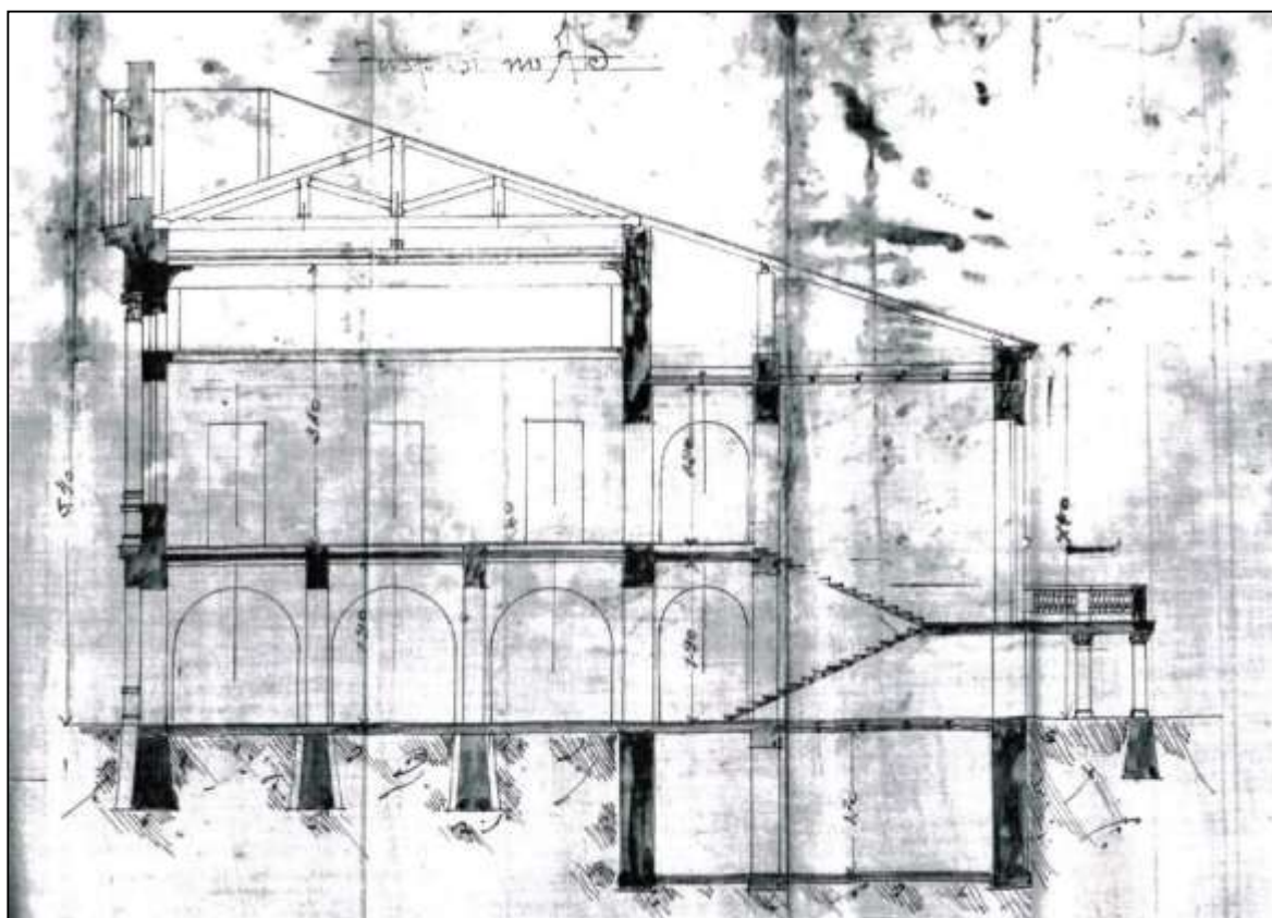
Фото 8. Поперечный разрез здания Общественного собрания. Арх. В.А. Соколовский, 1913 г. Из фондов ГАКК
