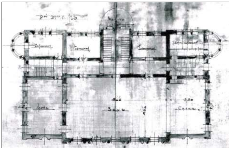
Фото 10. План второго этажа здания Общественного собрания. Арх. В.А. Соколовский, 1913 г. Из фондов ГАКК
