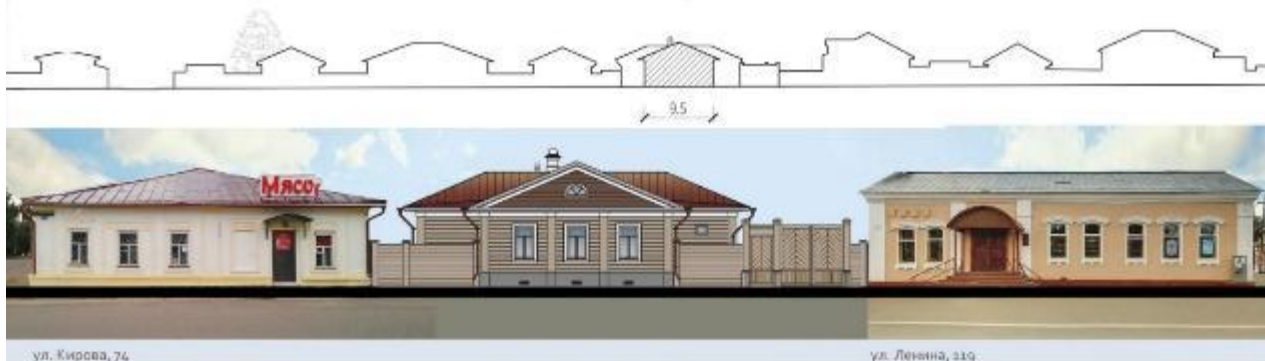
Вариант 1. Главный фасад в осях 1-4
